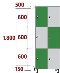
FM-40/2 COD: 53134 93kg · 0,71m 3
