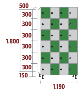
FB-30/4 COD: 53163 180kg · 1,07m 3
