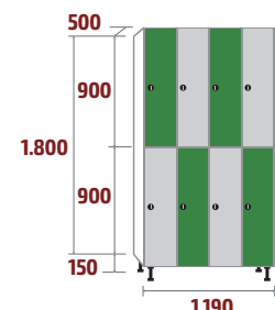
FT-30/4 COD: 53122 136,85kg · 1,07m 3
