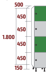
FC-30/1 COD: 53021 50kg · 0,27m 3
