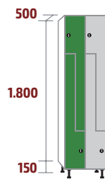
FL-30/2 COD: 53181 92kg · 0,54m 3
