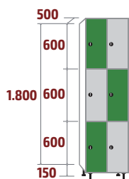
FM-30/2 COD: 53131 80kg · 0,54m 3
