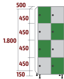
FC-40/2 COD: 53144 99kg · 0,71m 3
