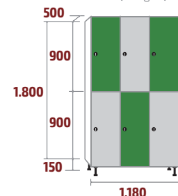
FT-40/3 COD: 53124 122,3kg · 1,06m 3
