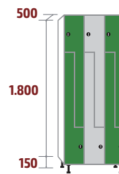
FL-30/3 COD: 53182 134kg · 0,81m 3
