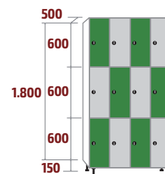
FM-30/4 COD: 53133 148kg · 1,07m 3
