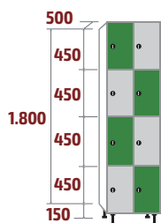
FC-30/2 COD: 53141 86kg · 0,54m 3
