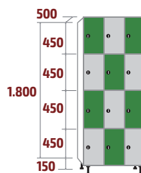
FC-30/3 COD: 53142 122kg · 0,81m 3
