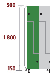
FL-40/2 COD: 53184 103kg · 0,71m 3
